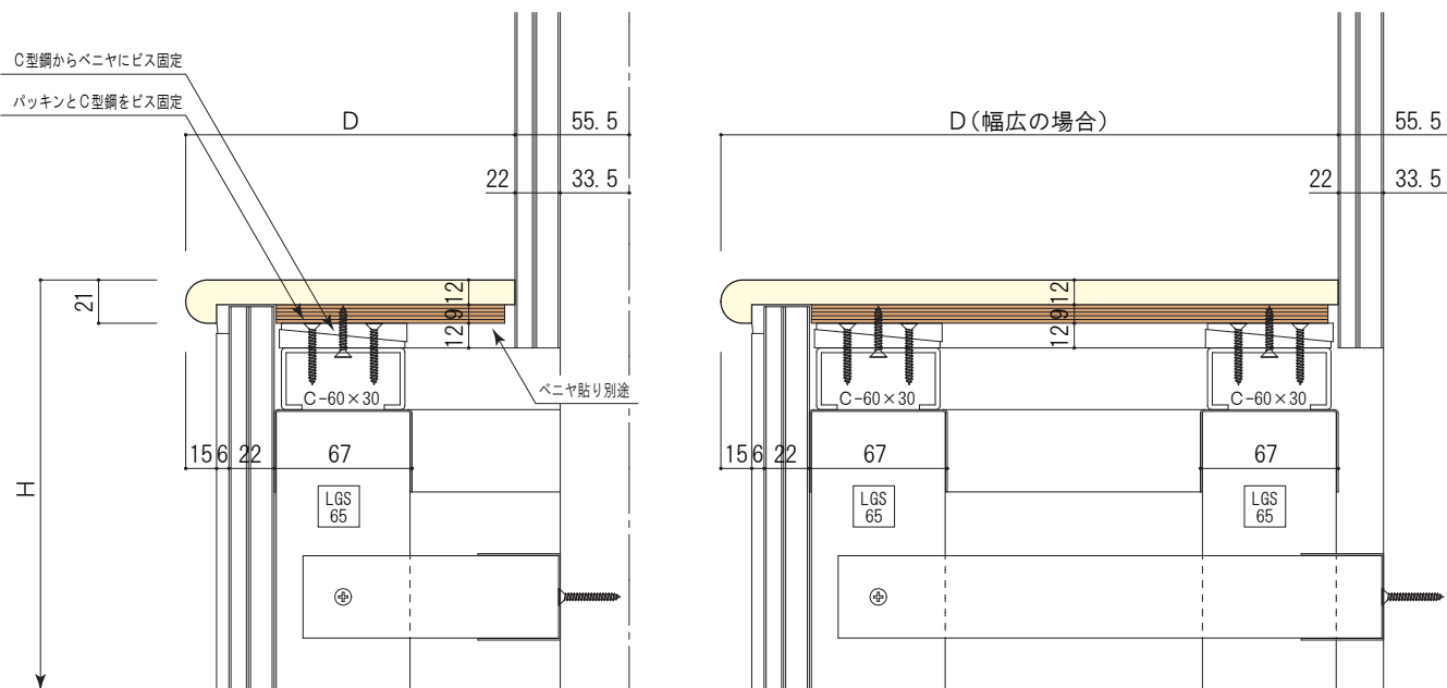
断面詳細図 (参考)
